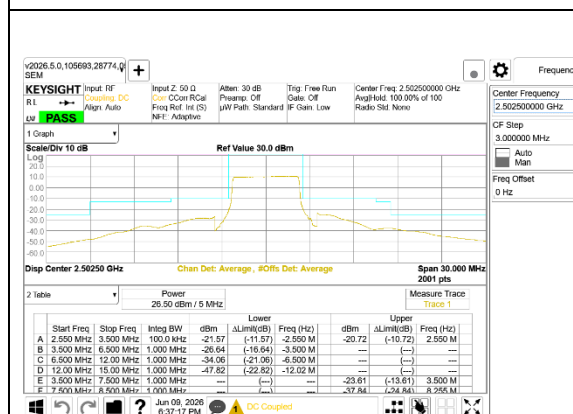
5G NR n7 5MHz BPSK Low Channel RB25-0
