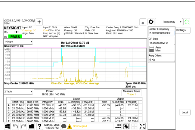
ULCA LTE B7 20MHz + 20MHz 16QAM Low Ch RB1-0 + RB1-99
