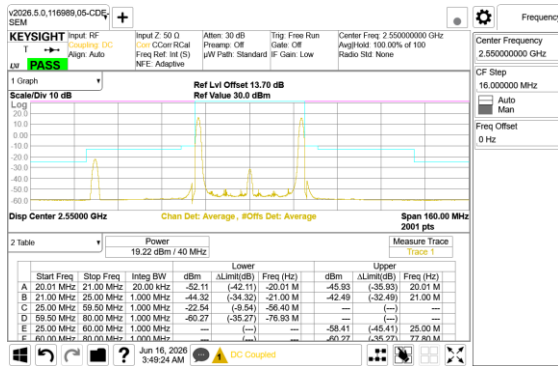
ULCA LTE B7 20MHz + 20MHz QPSK High Ch RB1-0 + RB1-99
