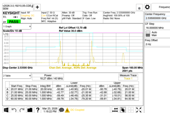
ULCA LTE B7 20MHz + 20MHz QPSK Mid Ch RB1-0 + RB1-99
