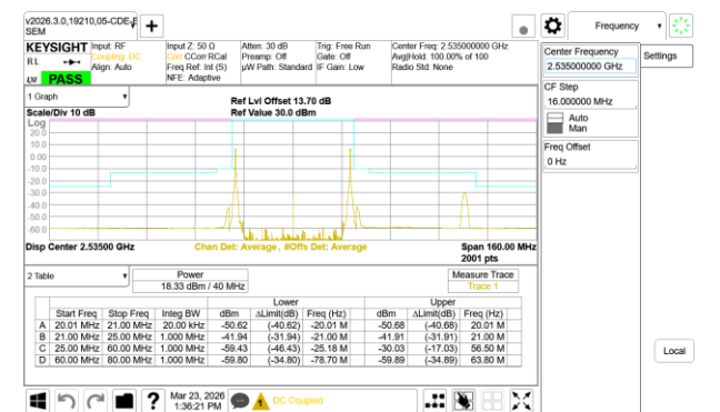
ULCA LTE B7 20MHz + 20MHz 16QAM Mid Ch RB1-0 + RB1-99
