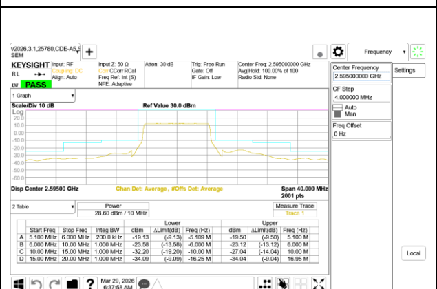
5G NR n41 10MHz BPSK Middle Channel RB24-0
