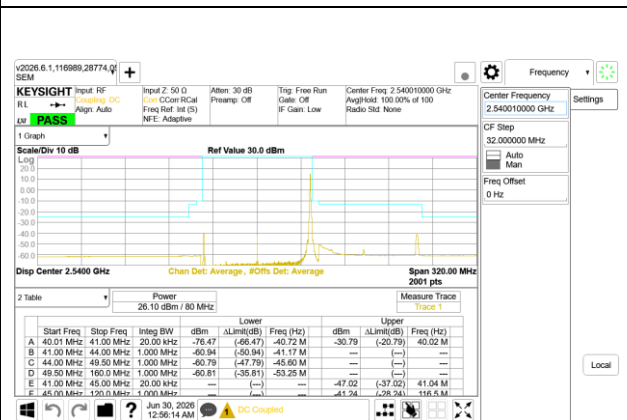
5G NR n41 80MHz BPSK Low Channel RB1-216
