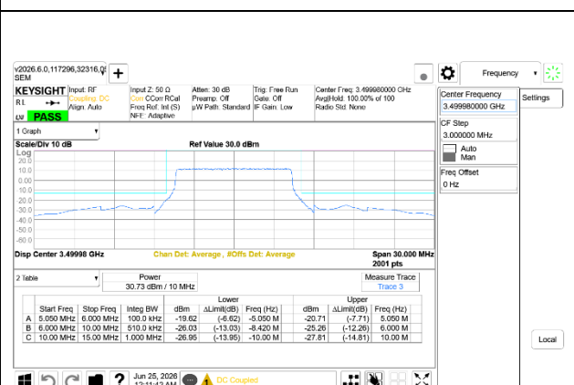
5G NR n77 10MHz BPSK Mid Channel RB24-0, Ant9+Ant8
