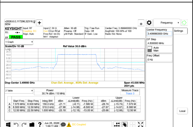
5G NR n77 15MHz BPSK Mid Channel RB36-0, Ant9+Ant8
