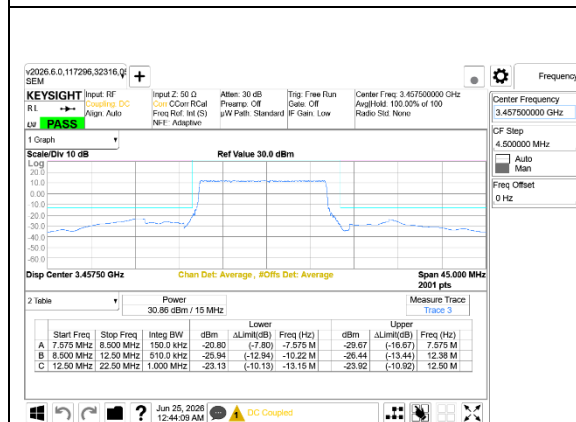
5G NR n77 15MHz BPSK Low Channel RB36-0, Ant9+Ant8
