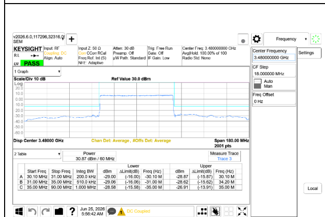
5G NR n77 60MHz BPSK Low Channel RB162-0, Ant9+Ant8
