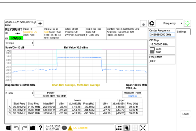
5G NR n77 60MHz BPSK Mid Channel RB162-0, Ant9+Ant8
