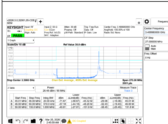
5G NR n77 90MHz BPSK Mid Channel RB1-244, Ant9+Ant8
