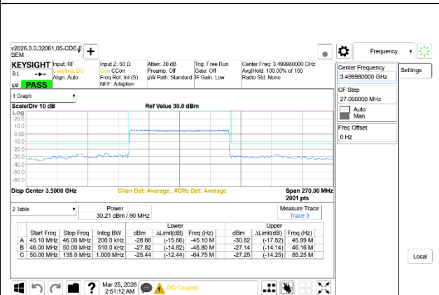
5G NR n77 90MHz BPSK Mid Channel RB243-0, Ant9+Ant8
