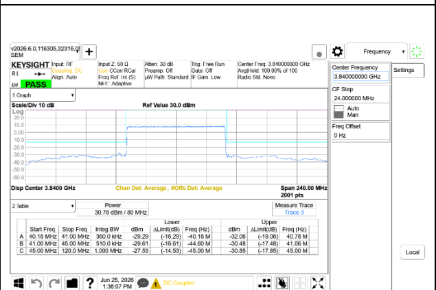
5G NR n77 80MHz BPSK Mid Channel RB216-0, Ant9+Ant8
