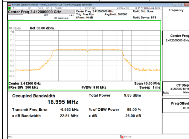
EHT20-mode - 2412 Channel - SU - ANT 3
