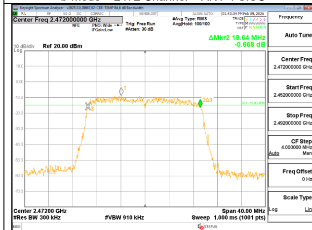
EHT20-mode – 2472 Channel – SU – ANT 3 SISO
