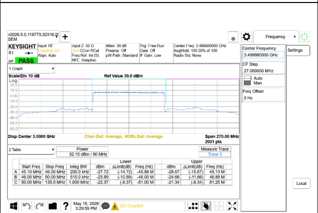
5G NR n77 90MHz BPSK Mid Channel RB243-0 Ant7+Ant8
