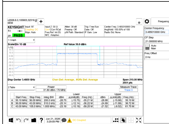
5G NR n77 70MHz BPSK Low Channel RB180-0 Ant7+Ant8
