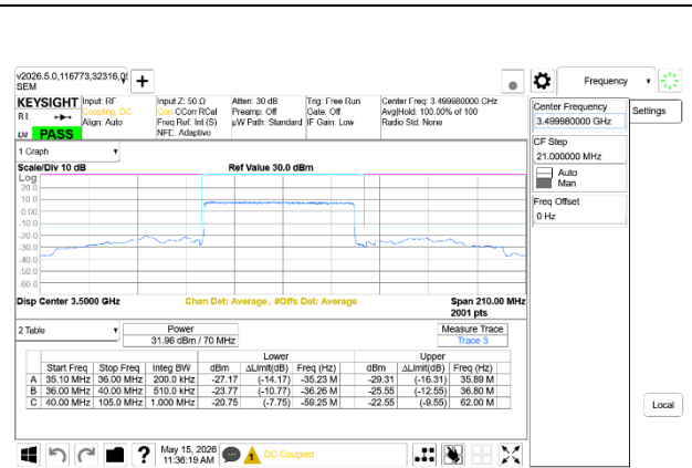
5G NR n77 70MHz BPSK Mid Channel RB180-0 Ant7+Ant8
