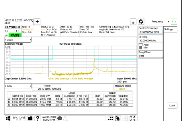
5G NR n77 100MHz BPSK Mid Channel RB1-272
