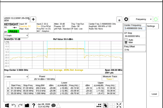
5G NR n77 100MHz BPSK Mid Channel RB270-0
