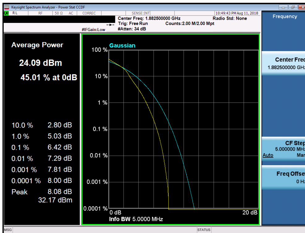
Plot 7-403. PAR Plot (Band 25 - 5.0MHz 16-QAM - RB Size 25)
