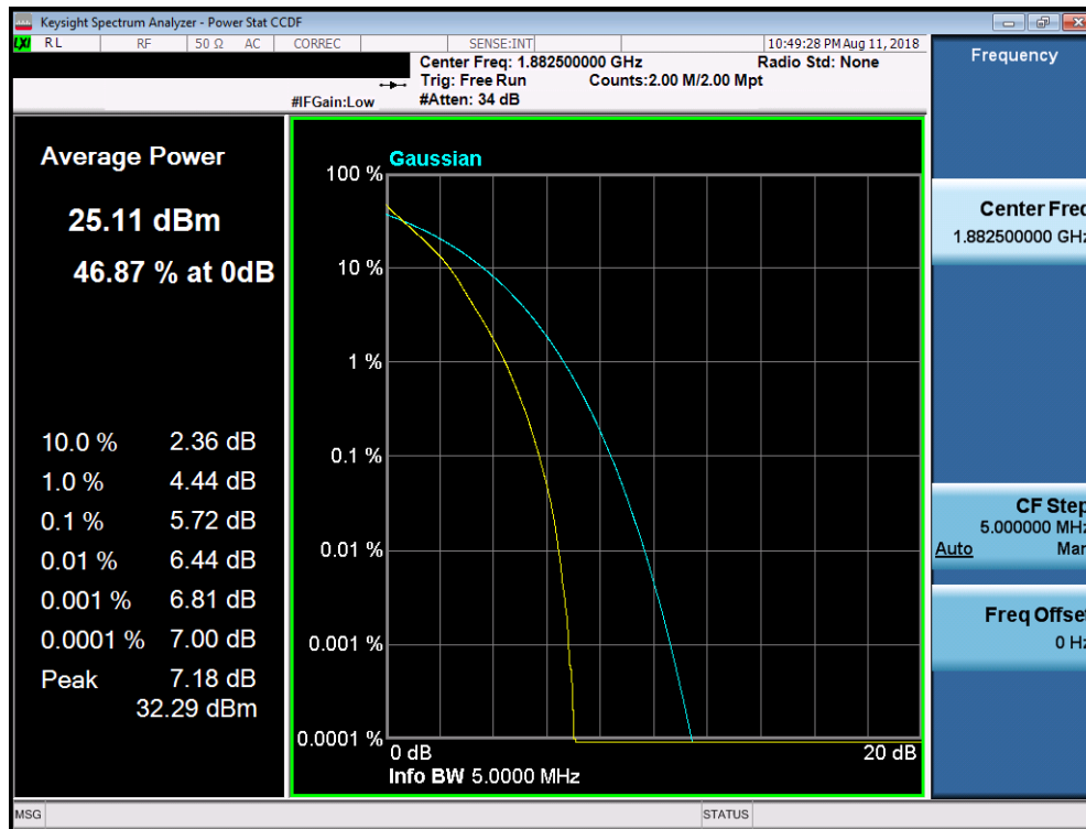
Plot 7-402. PAR Plot (Band 25 - 5.0MHz QPSK - RB Size 25)
