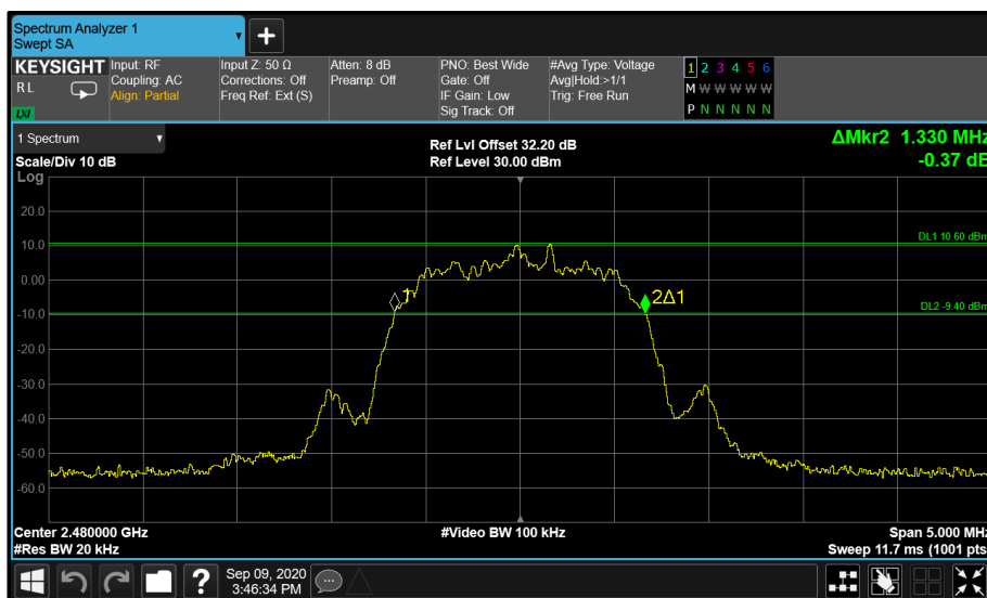
Figure 57 - Core 1 \pi/4 DQPSK 2480 MHz (CH78)
