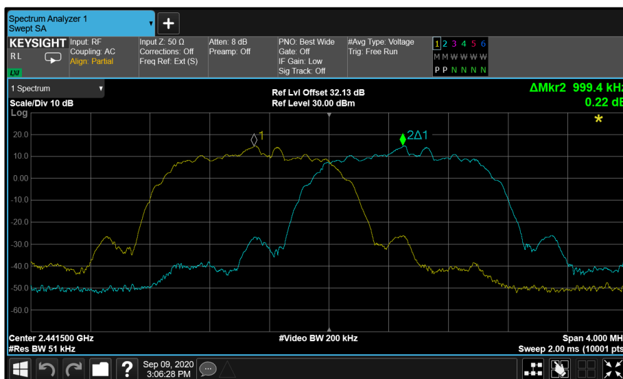
Figure 7 - \pi/4 DQPSK - 2441 MHz (CH 39)
