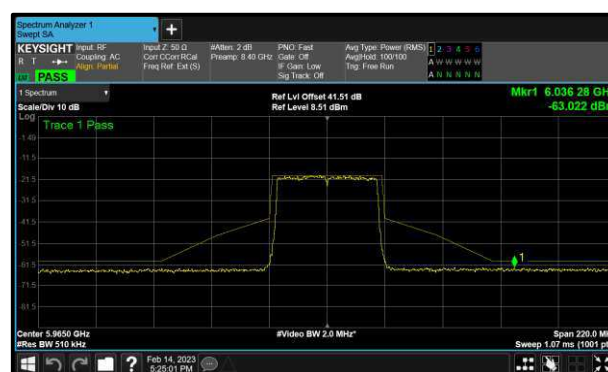
Figure 122 – A (Core 0) 802.11ax HE40 SU 5965 MHz (CH3)
