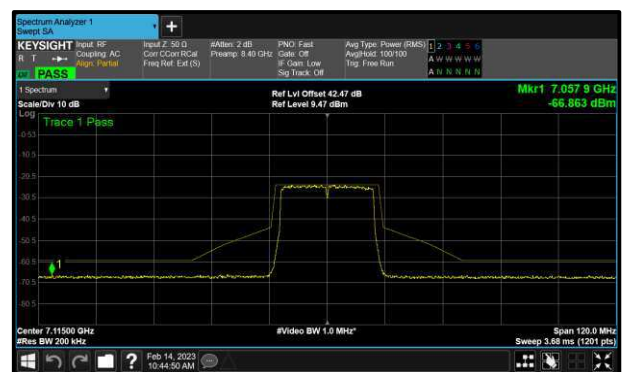
Figure 108 – A (Core 0) 802.11ax HE20 SU 7115 MHz (CH233)
