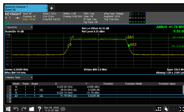
Figure 28 - 802.11ax HE40 SU Maximum 99% OBW
