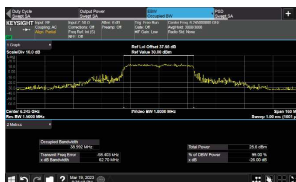
Figure 28 - 802.11ax HE40 SU Maximum 99% dB OBW
