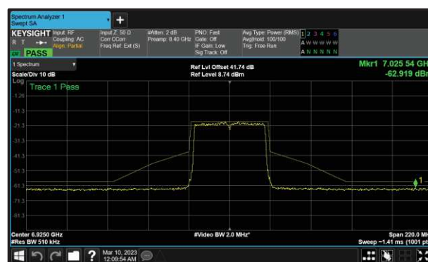
Figure 141 - C (Core 1) 802.11ax HE40 SU 6925 MHz (CH195)
