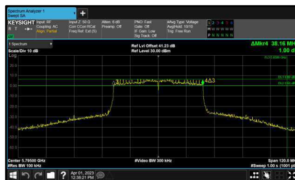
Figure 171 - 802.11ax HE40 SU Maximum 6 dB EBW
