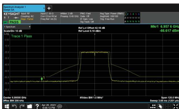
Figure 150 - A (Core 0) 802.11ax HE20 SU 6995 MHz (CH209)
