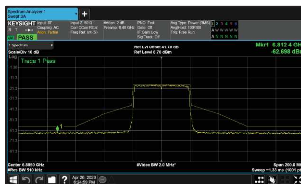
Figure 151 - B (Core 1) 802.11ax HE40 SU 6885 MHz (CH187)
