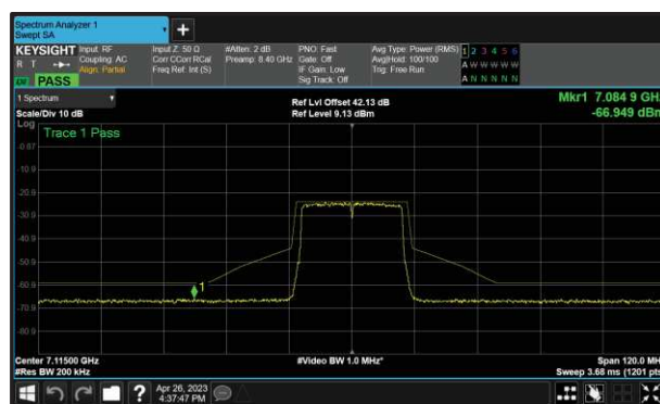
Figure 143 - A (Core 0) 802.11ax HE20 SU 7115 MHz (CH233)
