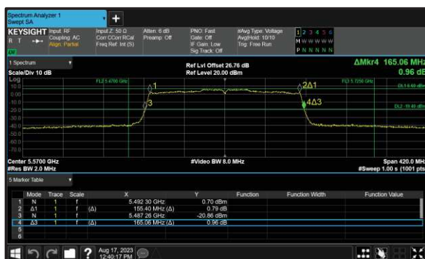
Figure 282 - 802.11ax HE160 SU Minimum 99% OBW
