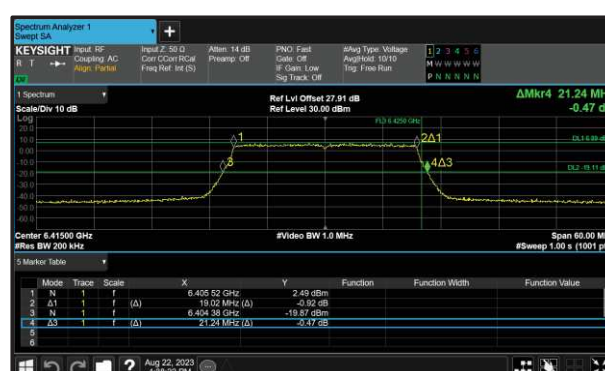
Figure 30 - 802.11ax HE20 SU SP Maximum 99% OBW
