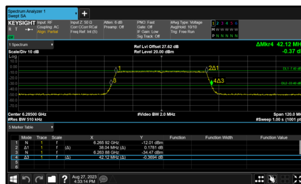
Figure 54 - 802.11ax HE40 SU LPI Maximum 99% OBW
