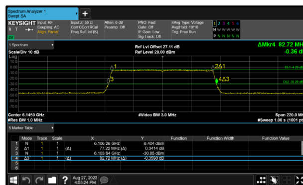
Figure 56 - 802.11ax HE80 SU LPI Maximum 99% OBW
