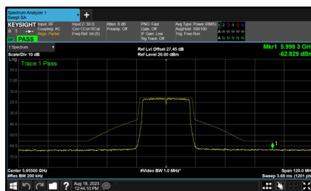
Figure 168 - A (Core 0) 802.11ax HE20 SU LPI 5955 MHz (CH1)
