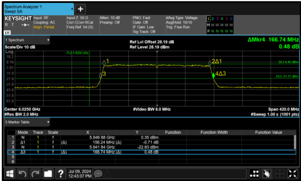
Figure 65 - 802.11ax HE160 SU LPI Minimum 99% OBW
