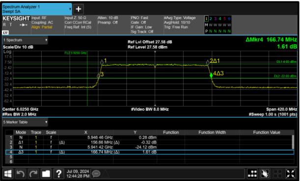
Figure 66 - 802.11ax HE160 SU LPI Maximum 99% OBW
