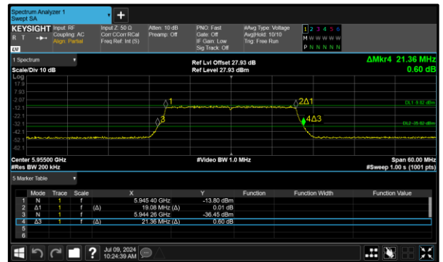
Figure 60 - 802.11ax HE20 SU LPI Maximum 99% OBW
