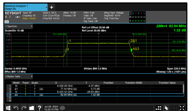
Figure 64 - 802.11ax HE80 SU LPI Maximum 99% OBW
