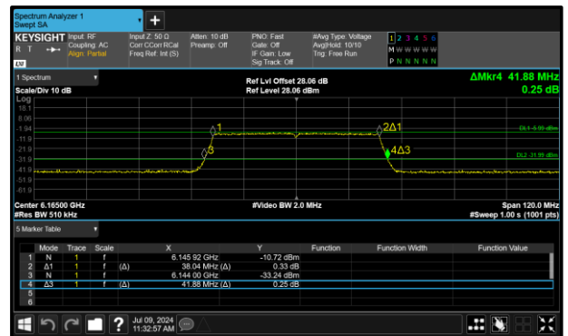
Figure 62 - 802.11ax HE40 SU LPI Maximum 99% OBW
