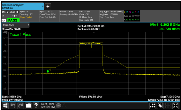
Figure 271 - A (Core 0) 802.11ax HE160 SU LPI 6505 MHz (CH111)
