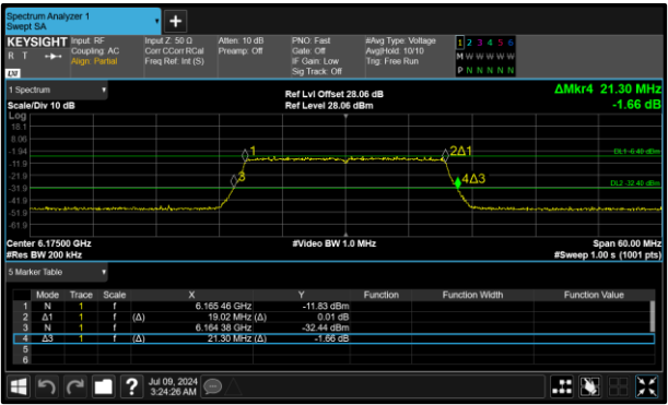
Figure 44 - 802.11ax HE20 SU LPI Maximum 99% OBW
