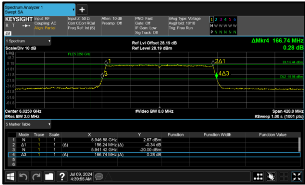
Figure 49 - 802.11ax HE160 SU LPI Minimum 99% OBW
