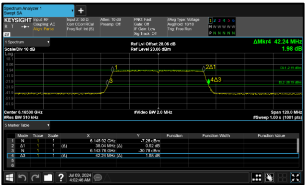
Figure 46 - 802.11ax HE40 SU LPI Maximum 99% OBW
