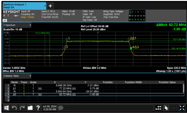
Figure 47 - 802.11ax HE80 SU LPI Minimum 99% OBW
