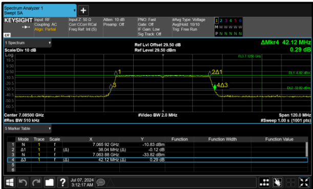
Figure 146 - 802.11ax HE40 SU LPI Maximum 26 dB EBW
