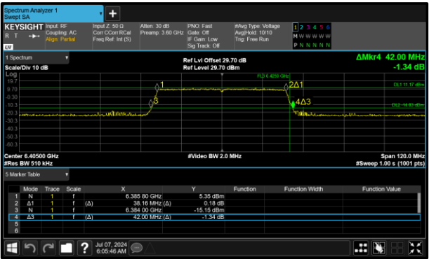
Figure 162 - 802.11ax HE40 SU SP Maximum 99% OBW
