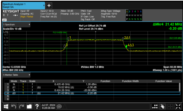
Figure 159 - 802.11ax HE20 SU SP Minimum 99% OBW
