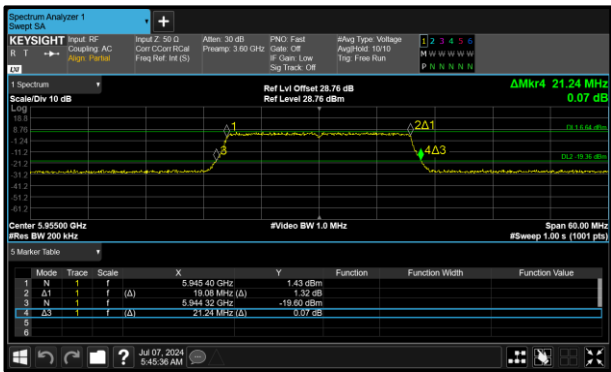
Figure 149 - 802.11ax HE20 SU SP Minimum 26 dB EBW
