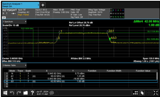
Figure 161 - 802.11ax HE40 SU SP Minimum 99% OBW
