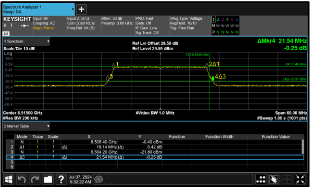
Figure 160 - 802.11ax HE20 SU SP Maximum 99% OBW
