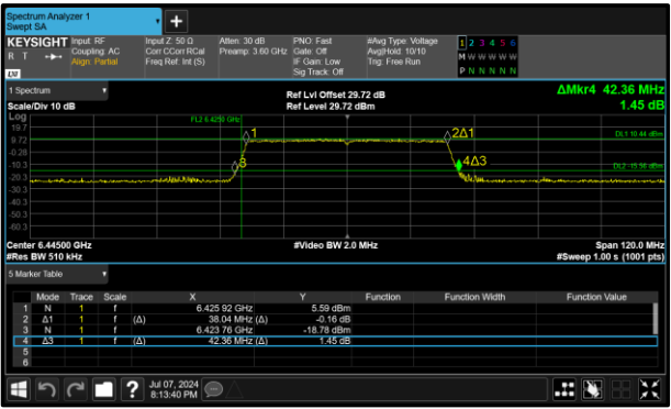
Figure 152 - 802.11ax HE40 SU SP Maximum 26 dB EBW
