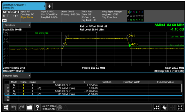
Figure 163 - 802.11ax HE80 SU SP Minimum 99% OBW
