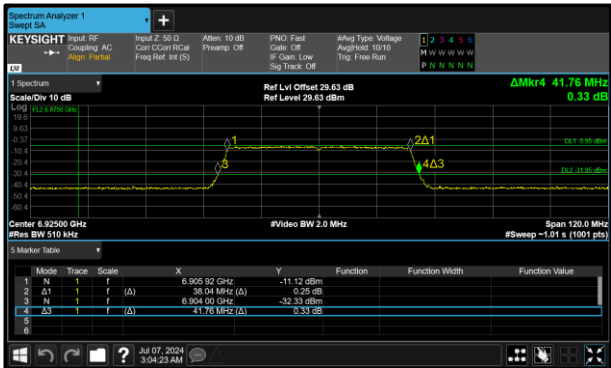
Figure 145 - 802.11ax HE40 SU LPI Minimum 26 dB EBW
