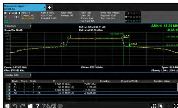
Figure 16 - 802.11ax HE40 SU Maximum 99% OBW
