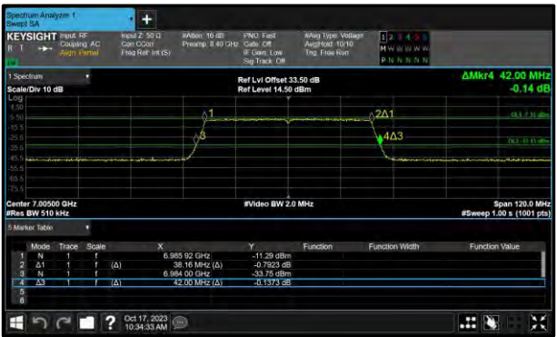
Figure 54 - 802.11ax HE40 SU Maximum 99% OBW
