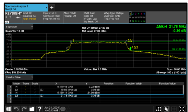
Figure 268 - 802.11ax HE20 SU Maximum 99% OBW
