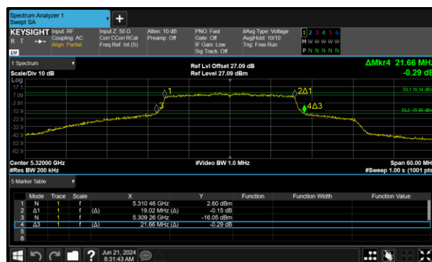
Figure 240 - 802.11ax HE20 SU Maximum 99% OBW
