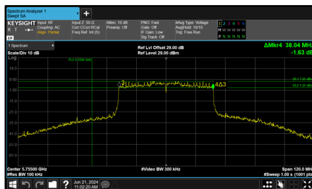
Figure 256 - 802.11ax HE40 SU Maximum 6 dB EBW
