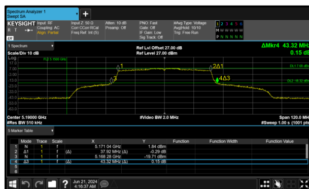
Figure 242 - 802.11ax HE40 SU Maximum 99% OBW
