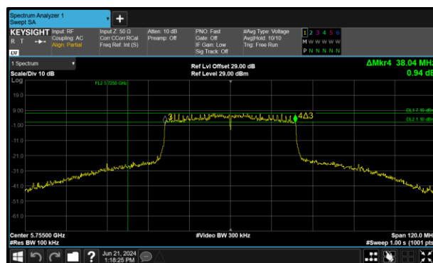
Figure 284 - 802.11ax HE40 SU Maximum 6 dB EBW
