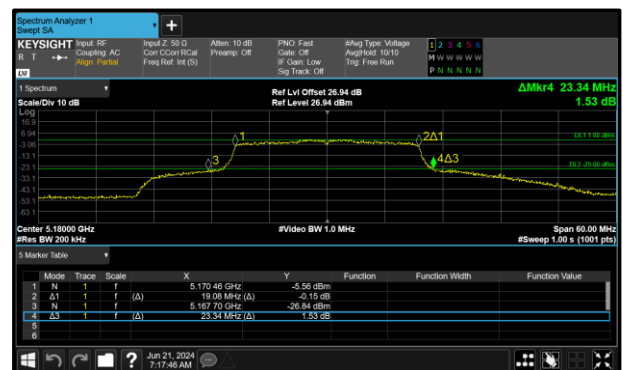
Figure 296 - 802.11ax HE20 SU Maximum 99% OBW
