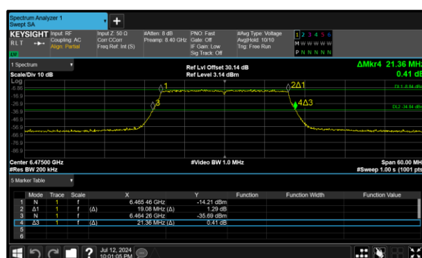
Figure 54 - 802.11ax HE20 SU LPI Maximum 99% OBW
