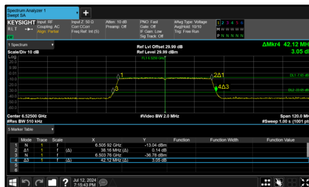
Figure 80 - 802.11ax HE40 SU LPI Maximum 99% OBW
