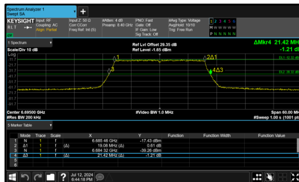
Figure 78 - 802.11ax HE20 SU LPI Maximum 99% OBW
