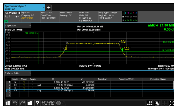
Figure 24 - 802.11ax HE20 SU LPI Maximum 99% OBW
