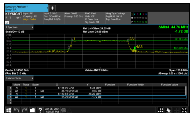
Figure 84 - 802.11ax HE40 SU SP Maximum 99% OBW
