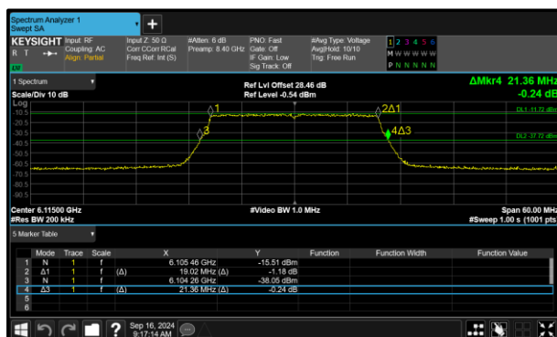
Figure 69 - 802.11ax HE20 SU VLP Minimum 99% OBW
