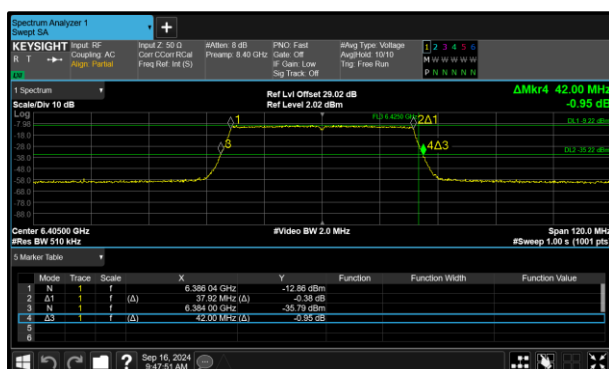
Figure 71 - 802.11ax HE40 SU VLP Minimum 99% OBW
