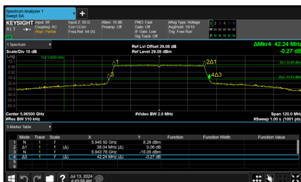
Figure 63 - 802.11ax HE40 SU SP Minimum 99% OBW
