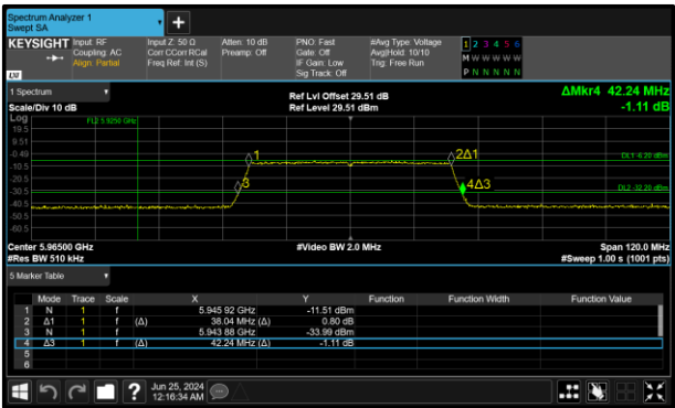
Figure 77 - 802.11ax HE40 SU LPI Minimum 99% OBW
