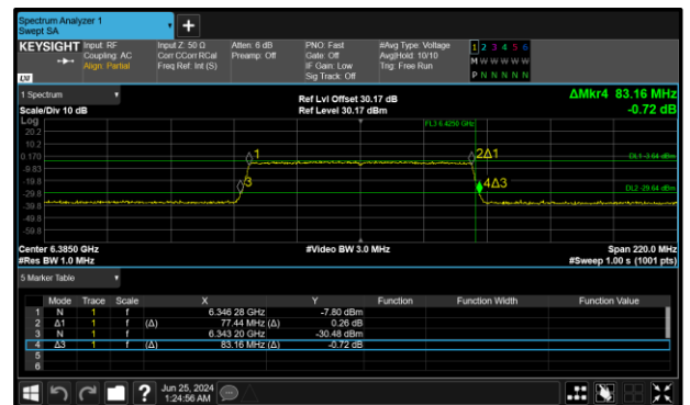
Figure 80 - 802.11ax HE80 SU LPI Maximum 99% OBW
