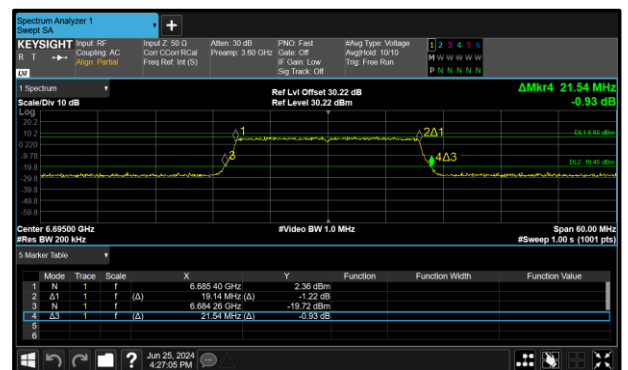
Figure 82 - 802.11ax HE20 SU SP Maximum 99% OBW
