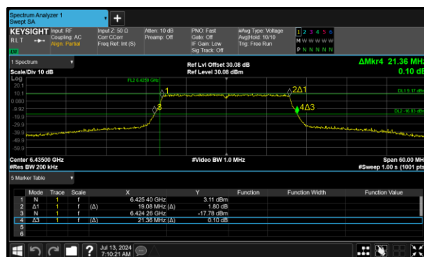
Figure 62 - 802.11ax HE20 SU SP Maximum 99% OBW
