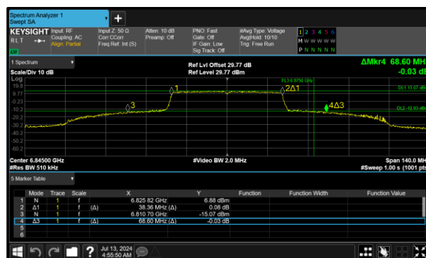
Figure 132 - 802.11ax HE40 SU SP Maximum 99% OBW
