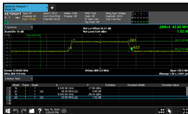
Figure 100 - 802.11ax HE40 SU VLP Maximum 99% OBW
