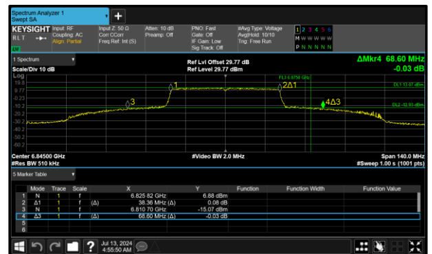
Figure 132 - 802.11ax HE40 SU SP Maximum 99% OBW
