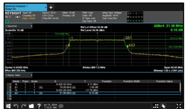
Figure 130 - 802.11ax HE20 SU SP Maximum 99% OBW
