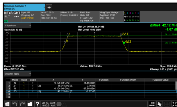
Figure 94 - 802.11ax HE40 SU VLP Maximum 26 dB EBW
