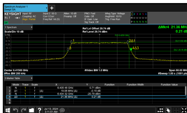
Figure 86 - 802.11ax HE20 SU SP Maximum 99% OBW
