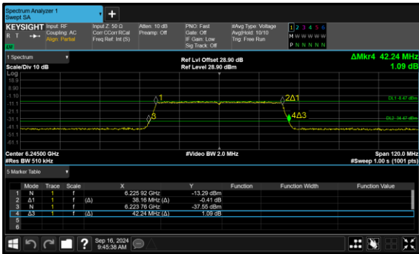
Figure 148 - 802.11ax HE40 SU VLP Maximum 99% OBW
