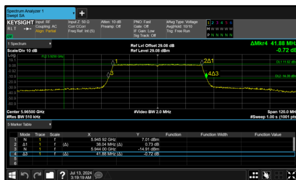
Figure 88 - 802.11ax HE40 SU SP Maximum 99% OBW
