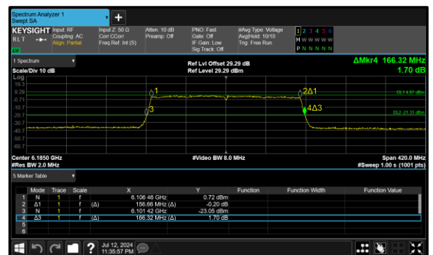
Figure 128 - 802.11ax HE160 SU LPI Maximum 99% OBW
