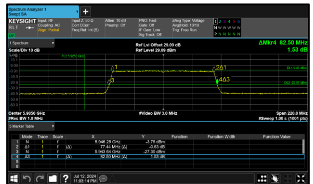
Figure 126 - 802.11ax HE80 SU LPI Maximum 99% OBW
