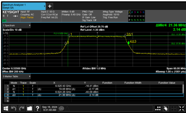
Figure 146 - 802.11ax HE20 SU VLP Maximum 99% OBW
