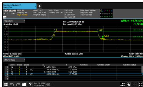
Figure 170 - 802.11ax HE40 SU SP Maximum 99% OBW
