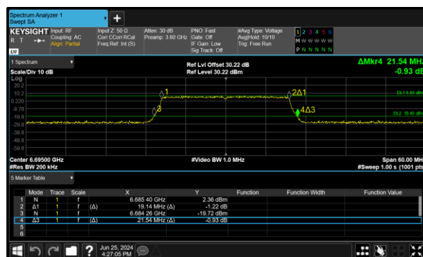
Figure 168 - 802.11ax HE20 SU SP Maximum 99% OBW
