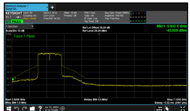
Figure 257 - B (Core 1) 802.11ax HE160 SU SP 6185 MHz (CH47)
