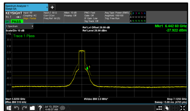
Figure 255 - A (Core 0) 802.11ax HE40 SU SP 6405 MHz (CH91)
