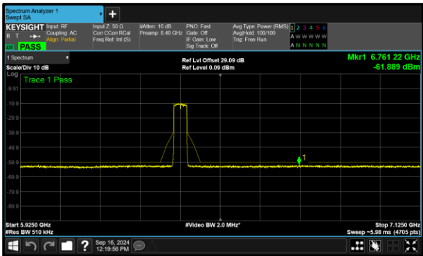
Figure 262 - B (Core 1) 802.11ax HE40 SU VLP 6405 MHz (CH91)
