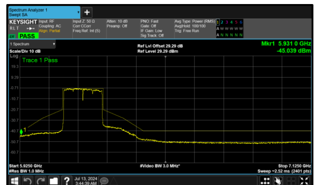
Figure 326 - B (Core 1) 802.11ax HE160 SU SP 6185 MHz (CH47)
