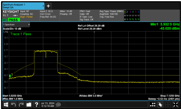
Figure 343 - B (Core 1) 802.11ax HE160 SU SP 6185 MHz (CH47)
