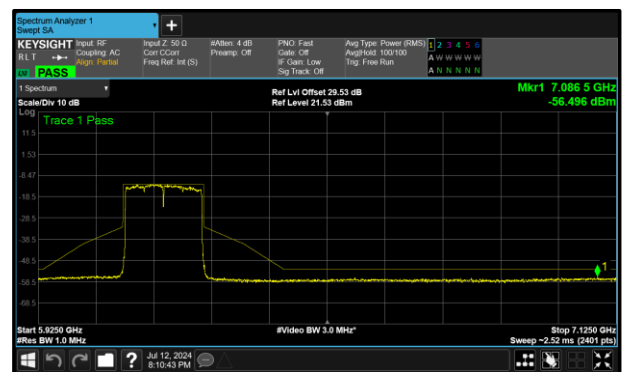
Figure 320 - A (Core 0) 802.11ax HE160 SU LPI 6185 MHz (CH47)
