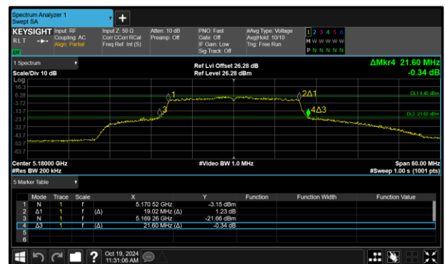
Figure 373 - 802.11ax HE20 SU Maximum 99% OBW
