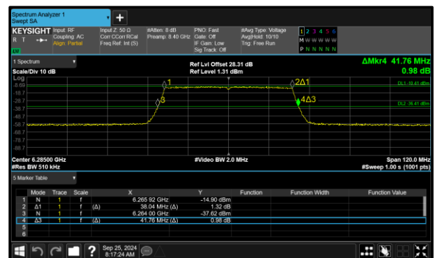
Figure 48 - 802.11ax HE40 SU VLP Maximum 99% OBW
