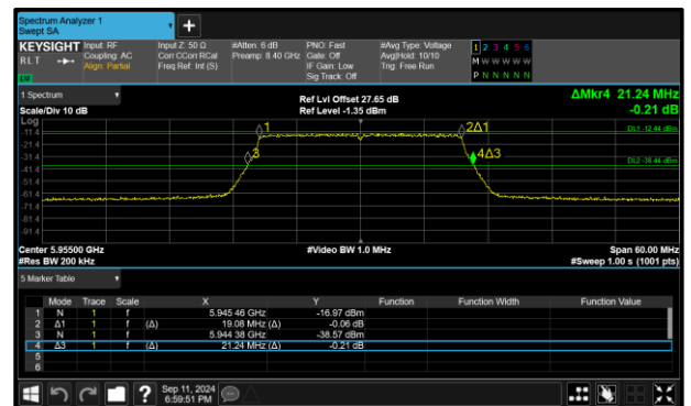
Figure 32 - 802.11ax HE20 SU LPI Maximum 99% OBW
