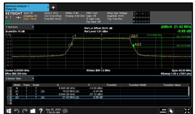
Figure 24 - 802.11ax HE20 SU VLP Maximum 99% OBW
