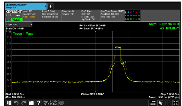
Figure 399 - A (Core 0) 802.11ax HE40 SU SP 6685 MHz (CH147)
