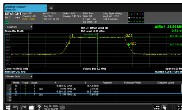
Figure 106 - 802.11ax HE20 SU LPI Maximum 26 dB EBW
