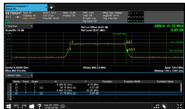
Figure 132 - 802.11ax HE40 SU LPI Maximum 99% OBW
