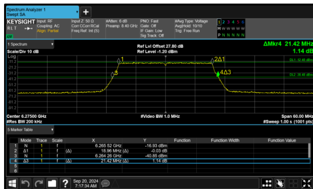
Figure 145 - 802.11ax HE20 SU VLP Minimum 99% OBW
