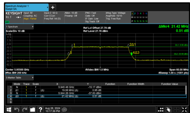
Figure 130 - 802.11ax HE20 SU LPI Maximum 99% OBW
