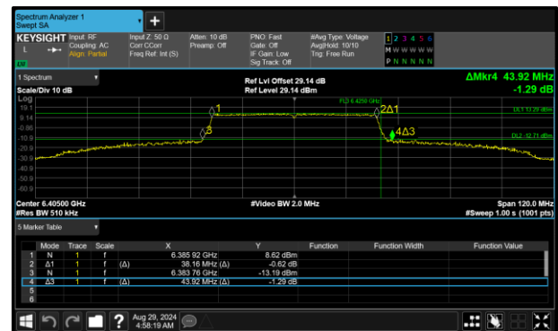
Figure 140 - 802.11ax HE40 SU SP Maximum 99% OBW
