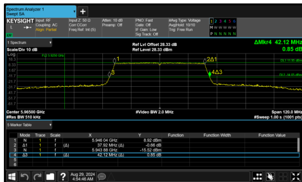
Figure 139 - 802.11ax HE40 SU SP Minimum 99% OBW
