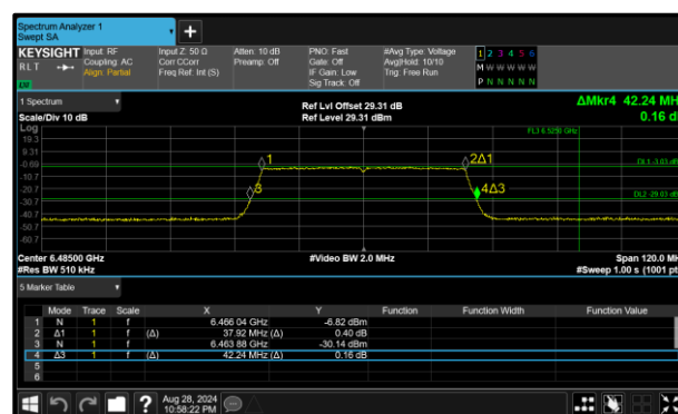
Figure 108 - 802.11ax HE40 SU LPI Maximum 26 dB EBW
