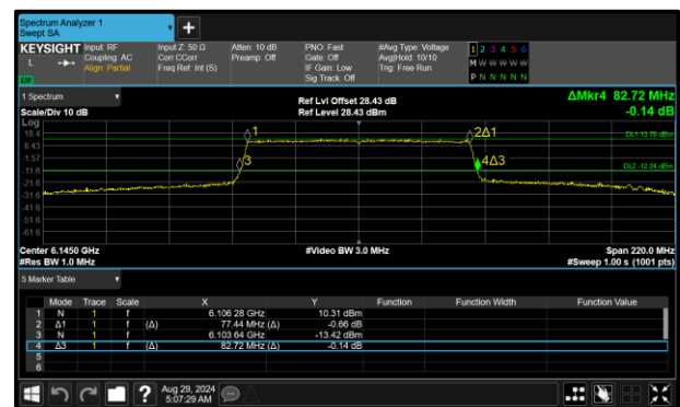
Figure 142 - 802.11ax HE80 SU SP Maximum 99% OBW
