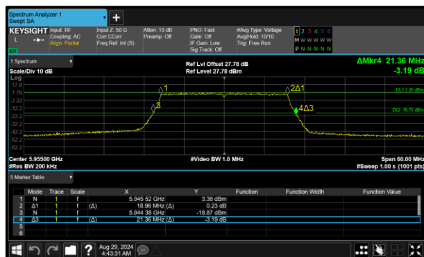
Figure 137 - 802.11ax HE20 SU SP Minimum 99% OBW
