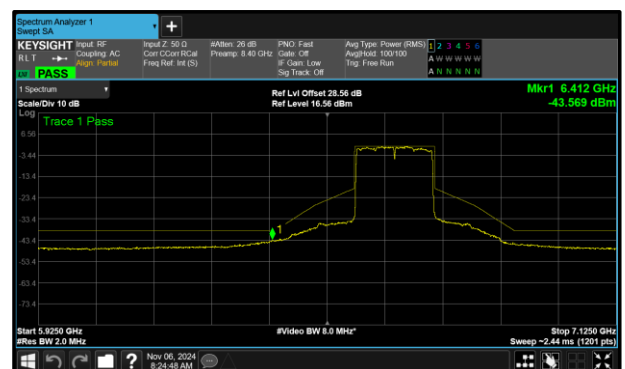
Figure 325 - A (Core 0) 802.11ax HE160 SU SP 6665 MHz (CH143)
