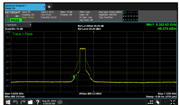
Figure 323 - A (Core 0) 802.11ax HE40 SU SP 6445 MHz (CH99)
