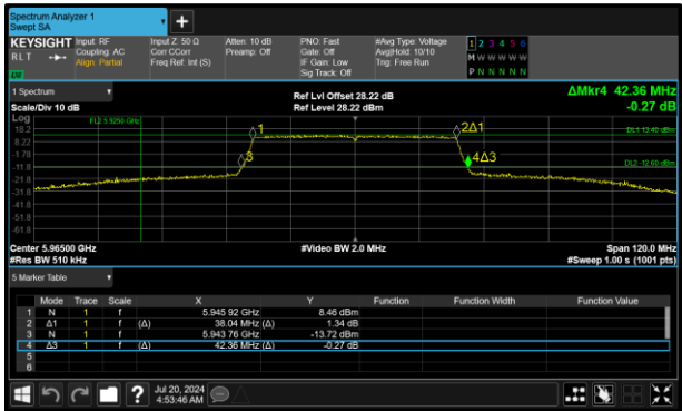
Figure 35 - 802.11ax HE40 SU SP Minimum 99% OBW
