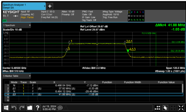
Figure 79 - 802.11ax HE40 SU LPI Minimum 99% OBW
