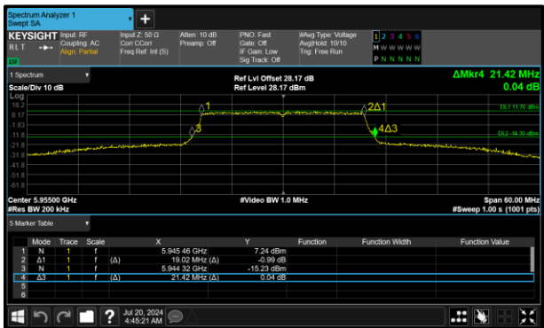
Figure 33 - 802.11ax HE20 SU SP Minimum 99% OBW
