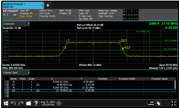
Figure 53 - 802.11ax HE20 SU VLP Minimum 99% OBW
