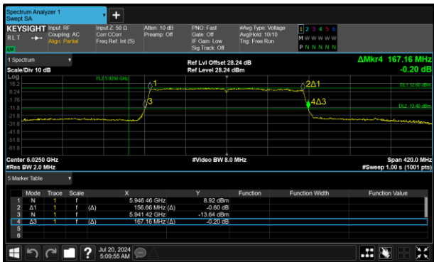
Figure 39 - 802.11ax HE160 SU SP Minimum 99% OBW
