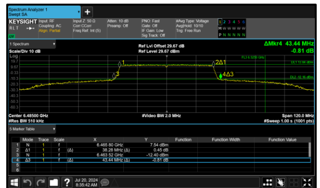
Figure 36 - 802.11ax HE40 SU SP Maximum 99% OBW
