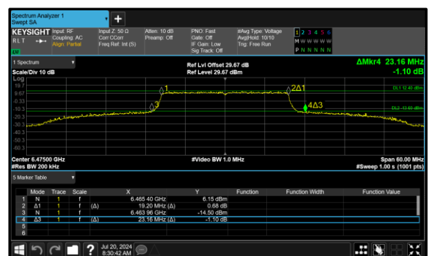
Figure 34 - 802.11ax HE20 SU SP Maximum 99% OBW
