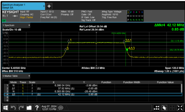
Figure 126 - 802.11ax HE40 SU LPI Minimum 99% OBW
