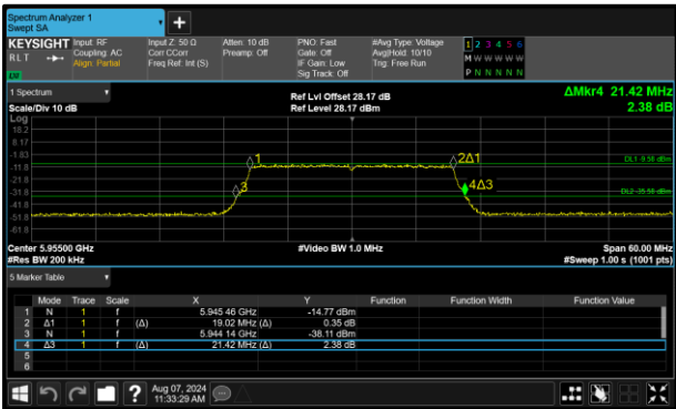
Figure 124 - 802.11ax HE20 SU LPI Minimum 99% OBW
