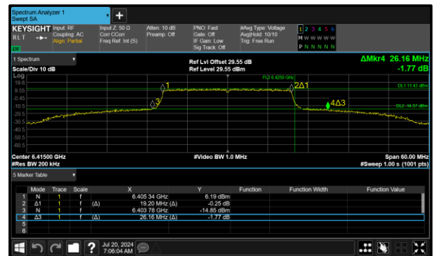
Figure 133 - 802.11ax HE20 SU SP Maximum 99% OBW
