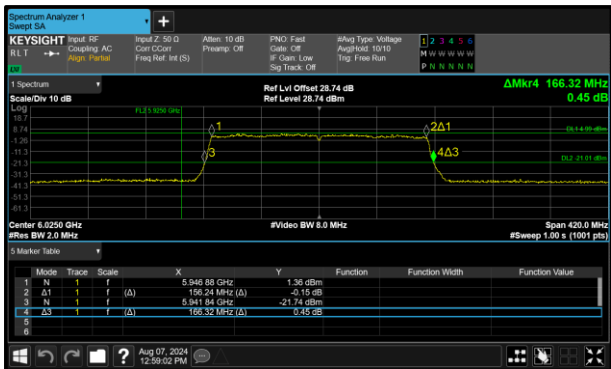
Figure 130 - 802.11ax HE160 SU LPI Minimum 99% OBW
