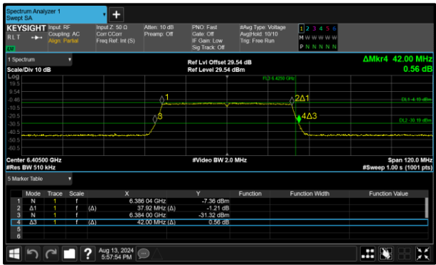
Figure 150 - 802.11ax HE40 SU VLP Minimum 99% OBW
