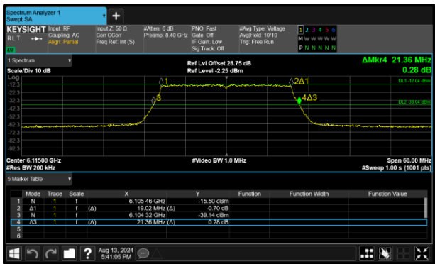
Figure 148 - 802.11ax HE20 SU VLP Minimum 99% OBW
