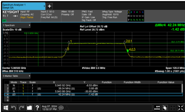
Figure 127 - 802.11ax HE40 SU LPI Maximum 99% OBW
