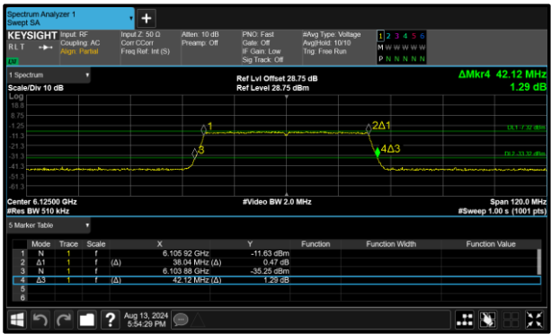
Figure 151 - 802.11ax HE40 SU VLP Maximum 99% OBW
