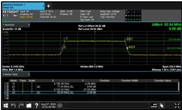
Figure 129 - 802.11ax HE80 SU LPI Maximum 99% OBW
