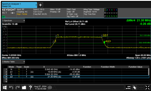
Figure 125 - 802.11ax HE20 SU LPI Maximum 99% OBW
