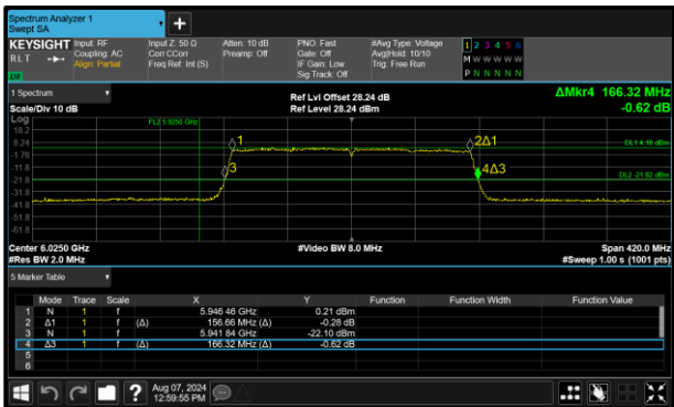
Figure 131 - 802.11ax HE160 SU LPI Maximum 99% OBW
