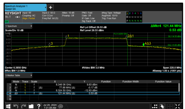
Figure 137 - 802.11ax HE80 SU SP Maximum 99% OBW
