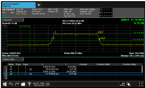
Figure 111 - 802.11ax HE40 SU LPI Minimum 26 dB OBW
