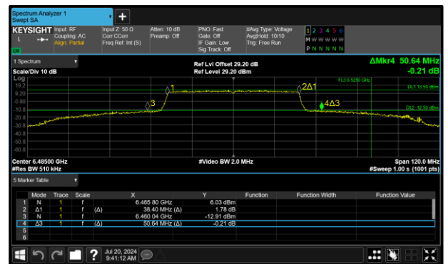
Figure 135 - 802.11ax HE40 SU SP Maximum 99% OBW
