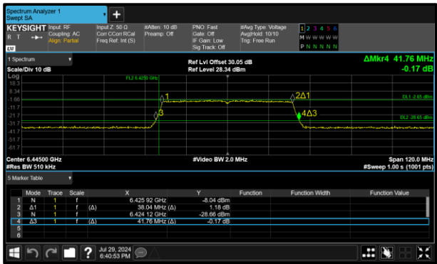
Figure 158 - 802.11ax HE40 SU LPI Minimum 26 dB OBW
