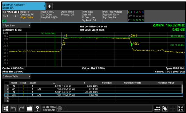
Figure 139 - 802.11ax HE160 SU SP Maximum 99% OBW
