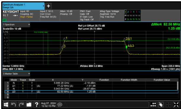
Figure 128 - 802.11ax HE80 SU LPI Minimum 99% OBW
