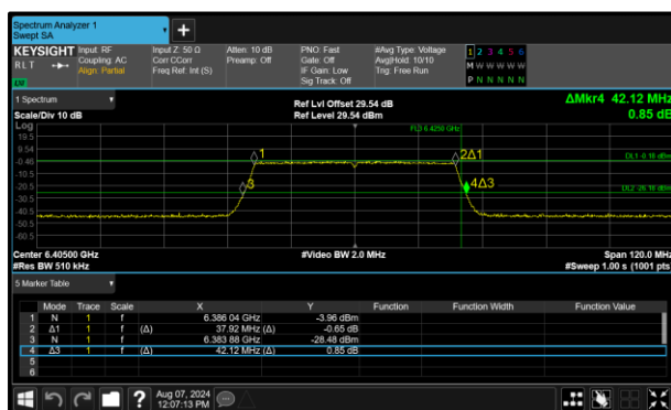
Figure 126 - 802.11ax HE40 SU LPI Minimum 99% OBW
