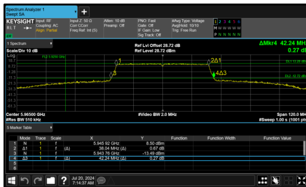
Figure 134 - 802.11ax HE40 SU SP Minimum 99% OBW
