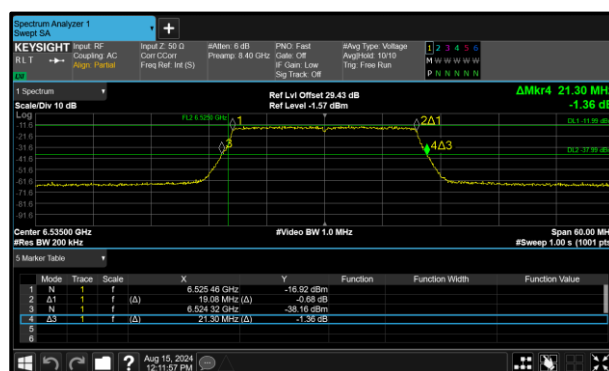
Figure 102 - 802.11ax HE20 SU VLP Maximum 99% OBW
