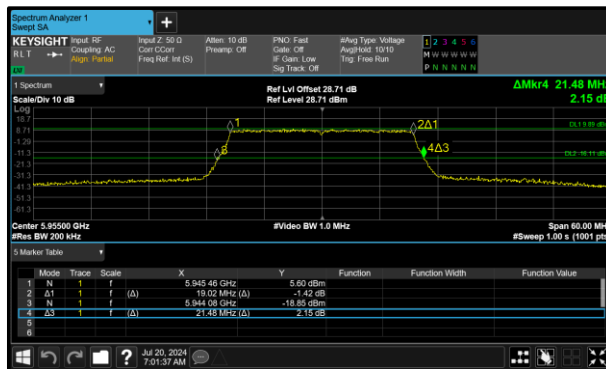
Figure 132 - 802.11ax HE20 SU SP Minimum 99% OBW
