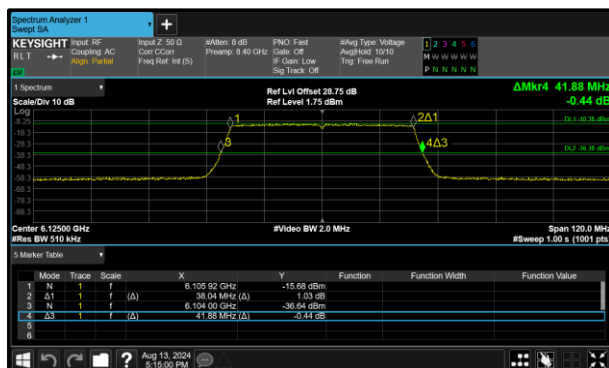
Figure 103 - 802.11ax HE40 SU VLP Minimum 99% OBW
