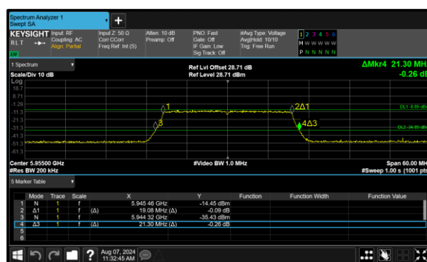
Figure 125 - 802.11ax HE20 SU LPI Maximum 99% OBW
