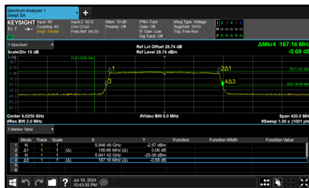
Figure 84 - 802.11ax HE160 SU LPI Maximum 99% OBW
