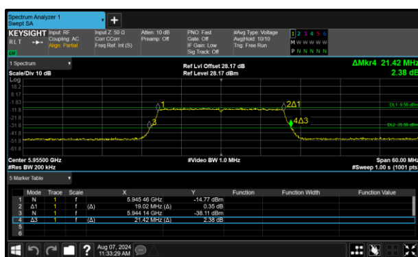
Figure 124 - 802.11ax HE20 SU LPI Minimum 99% OBW
