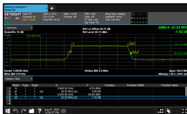
Figure 127 - 802.11ax HE40 SU LPI Maximum 99% OBW
