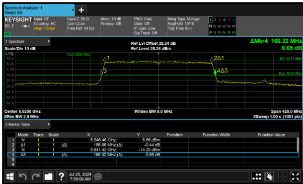
Figure 139 - 802.11ax HE160 SU SP Maximum 99% OBW
