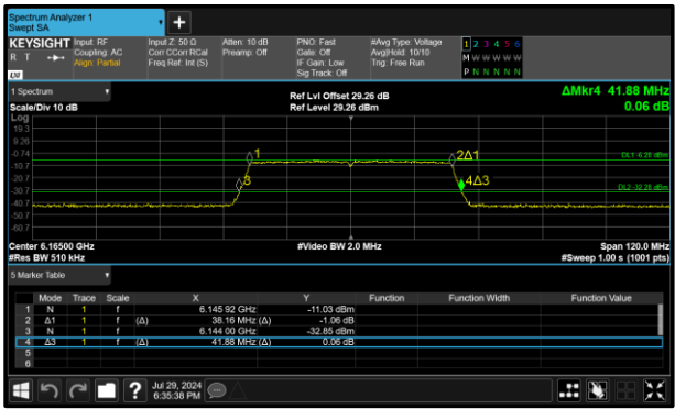
Figure 173 - 802.11ax HE40 SU LPI Maximum 99% OBW
