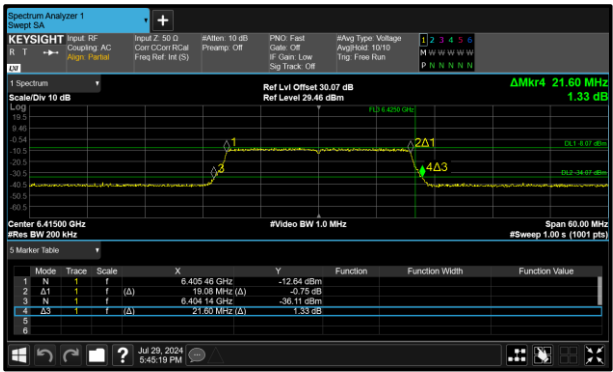
Figure 171 - 802.11ax HE20 SU LPI Maximum 99% OBW
