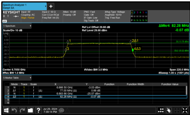
Figure 174 - 802.11ax HE80 SU LPI Minimum 99% OBW
