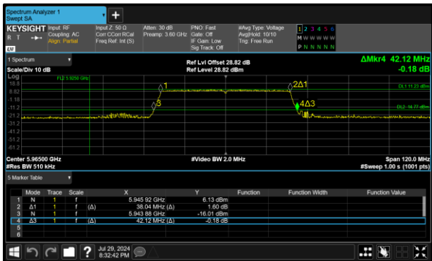
Figure 178 - 802.11ax HE40 SU SP Minimum 99% OBW
