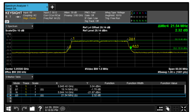
Figure 177 - 802.11ax HE20 SU SP Maximum 99% OBW
