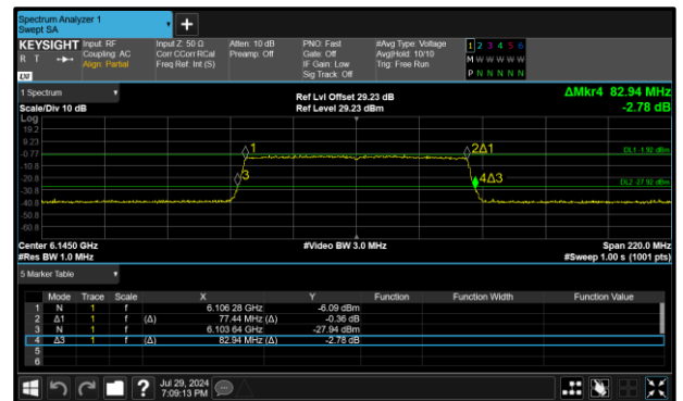
Figure 175 - 802.11ax HE80 SU LPI Maximum 99% OBW
