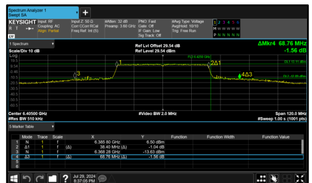
Figure 179 - 802.11ax HE40 SU SP Maximum 99% OBW
