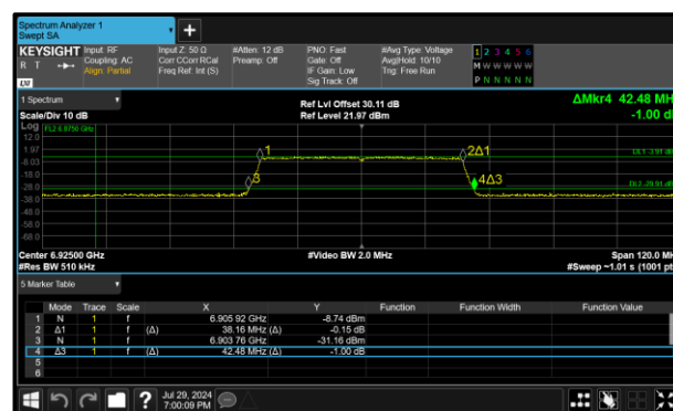
Figure 159 - 802.11ax HE40 SU LPI Maximum 26 dB OBW
