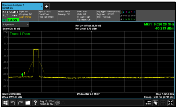
Figure 343 - A(Core 0) 802.11ax HE40 SU VLP 6125 MHz (CH35)
