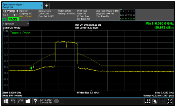
Figure 309 - A (Core 0) 802.11ax HE160 SU LPI 6345 MHz (CH79)
