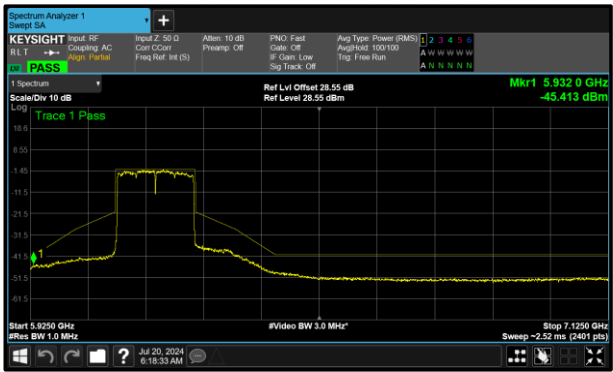
Figure 338 - B (Core 1) 802.11ax HE160 SU SP 6185 MHz (CH47)
