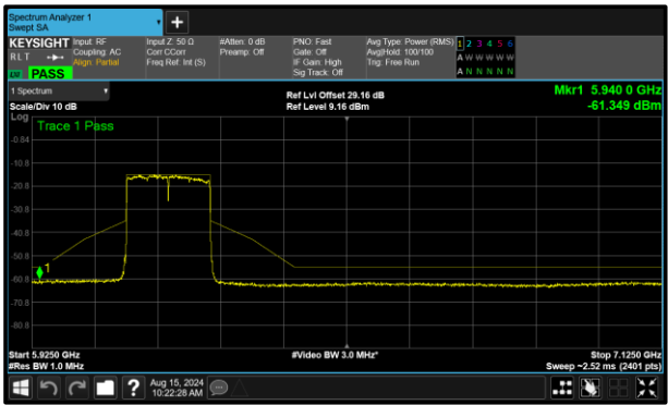
Figure 345 - A(Core 0) 802.11ax HE160 SU VLP 6185 MHz (CH47)
