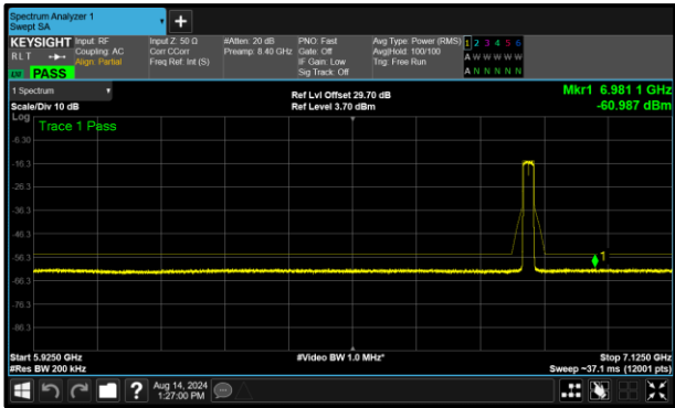
Figure 322 – A (Core 0) 802.11ax HE20 SU VLP 6855 MHz (CH181)
