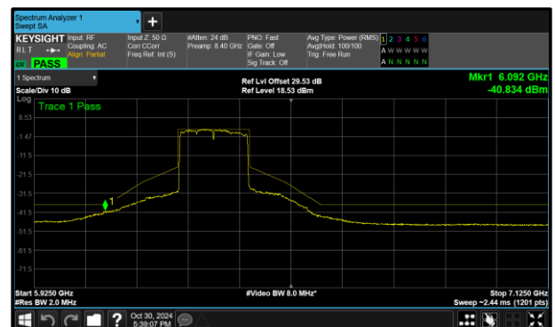
Figure 338 - A (Core 0) 802.11ax HE160 SU SP 6345 MHz (CH79)
